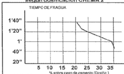
Diagrama N° 2 Tiempos de fragua en mortero según dosificación de CHEMA 2
